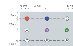
アルミプレートの温度測定位置
