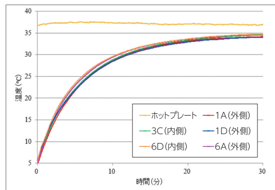
【図1】アルミプレート使用あり(2段タイプ※1)
