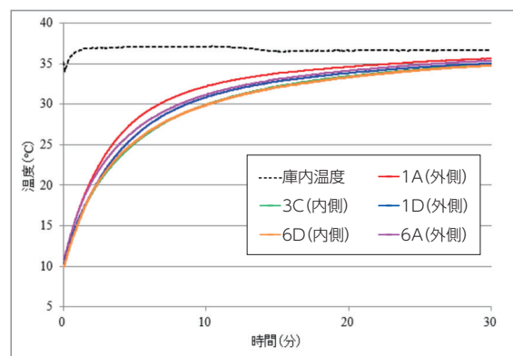
【図4】アルミプレート使用あり(2段タイプ※1)
