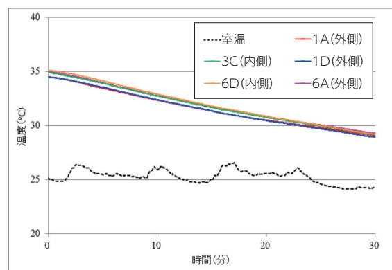
【図7】アルミプレート使用あり(2段タイプ※1)
